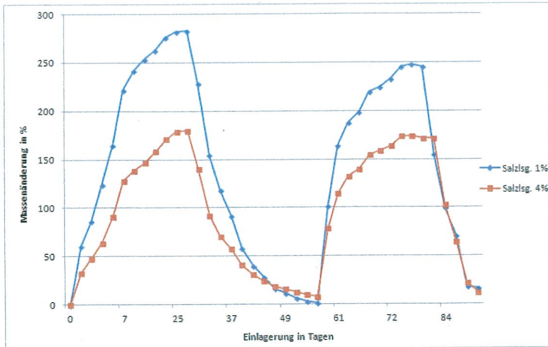
Bild A1: Massenänderung des Quellbandes bei Einlagerung in 1 %iger bzw. 4 %iger Salzlösung
